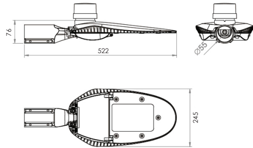
Outer Dimensions _____ Unit:mm
